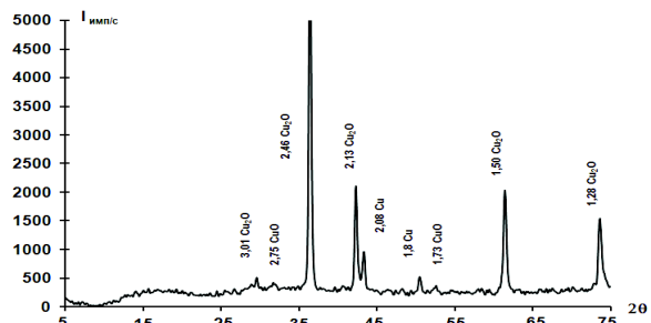
Рис. 6. – Рентгеноструктурная дифрактограмма полученного осадка
