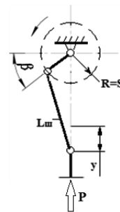
Рис. 2. – Геометричні характеристики кривошипно-шатунного привода: R – довжина кривошипа, що відповідає амплітуді коливань S ; L_{ш} – довжина шатуна; \beta – поточний кут повороту кривошипа; y – сумарний шлях, пройдений системою за один оберт кривошипа
