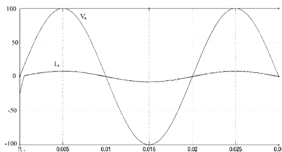
Рис. 5 – Временные диаграммы напряжения и тока фазы А.
