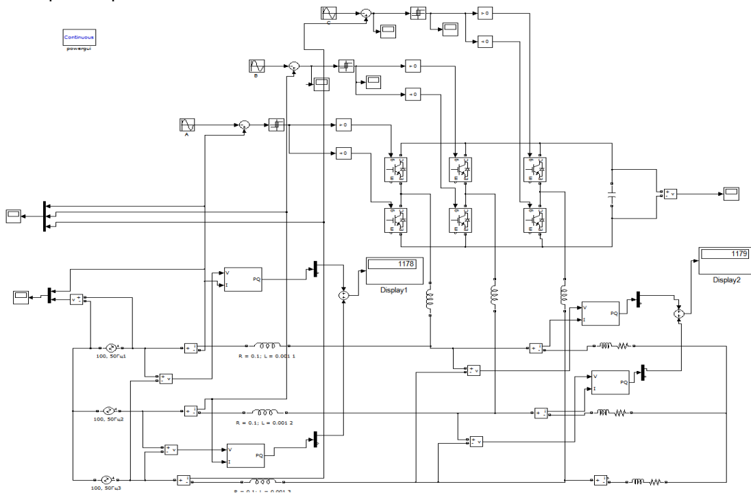
Рис. 2 – Визуальная модель системы электропитания с активным фильтром
