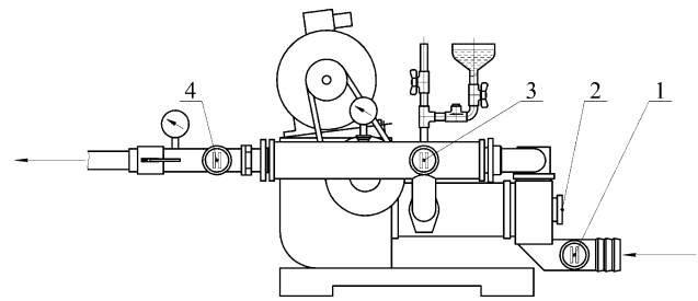
Рис. 5 – Схема встановлення тензометричних датчиків: 1 – усмоктувальний патрубок; 2 – усмоктувальна робоча камера; 3 – робоча камера компенсатора; 4 – нагнітальний патрубок
