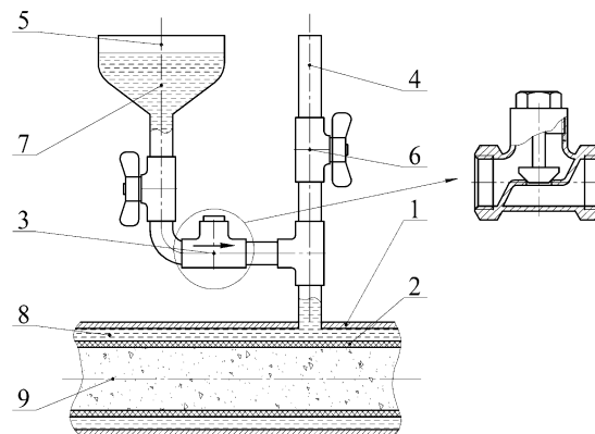
Рис. 2 – Пристрій для автоматичного поповнення робочої рідини: 1 – корпус гідравлічного компенсатора; 2 – трубчаста гумотканинна діафрагма; 3 – зворотний клапан; 4 – трубка для випуску повітря; 5 – місткість для робочої рідини; 6, 7 – шарові крани; 8 – робоча камера компенсатора; 9 – магістраль із розчинною сумішшю
