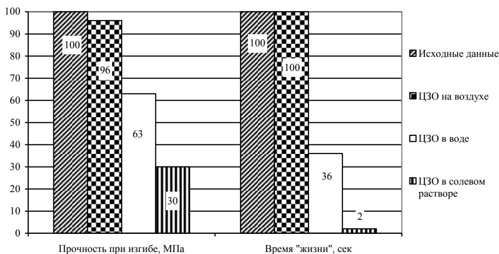
Рис. 1 – Потеря прочностных свойств асфальтобетона (в %) под влиянием ЦЗО (Исходное значение принято за 100 %)
