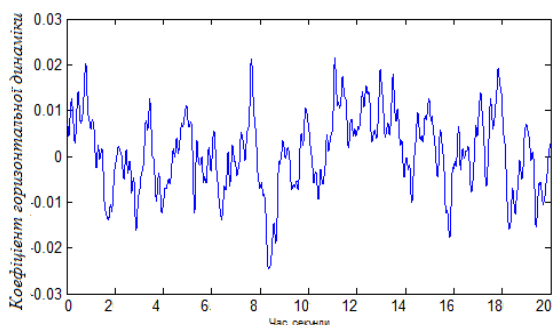
Рис. 3 – Осцилограма зміни коефіцієнту горизонтальної динаміки при швидкості 100 км/год на прямій дільниці колії
