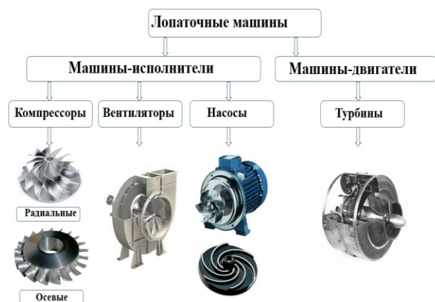
Рис. 5 - Типы лопаточных машин
