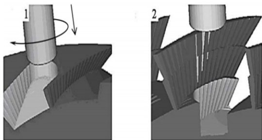
Рис. 8 - Плу́нжерное фрезерование межлопаточного канала [18]: 1 – межлопаточный канал в начале обработки; 2 – межлопаточный канал в конце обработки
