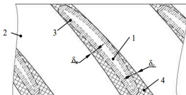
Рис. 9 - Погрешность формообразования межлопаточных каналов кольцевым инструментом: 1 – теоретический профиль пера лопатки; 2 – удаленный объем материала межлопаточного канала; 3 – слой припуска; 4 – слой металла, образованный из-за погрешности формообразования.
