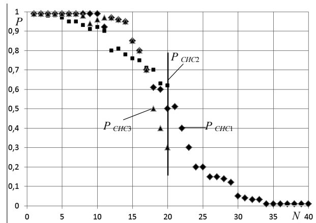
Рис. 2 – Вигляд розподілів значень ймовірності безвідмовної роботи при моделюванні поведінки технічної системи
