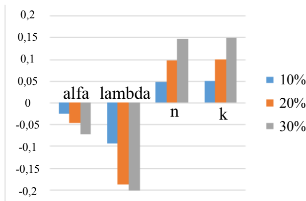
Рис. 2 – Относительное влияние параметров плана на информационное содержание модели компонент дисперсий (случайной) (n = 100; k = 10; \alpha = 0,05; \lambda = 1)
