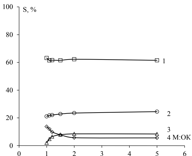
Рис. 5 – Вплив співвідношення реагентів на селективності утворення Мац(1), АК (2), МАкр (3), АЦ (4) у присутності каталізатора K_2 . Час контакту 8с; температура процесу 350 °С
