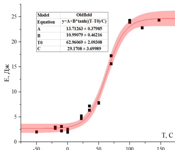
Рис. 2 – Результати випробувань стандартних зразків Шарпі та апроксимація кривої в'язко-крихкого переходу за функцією Олدفілда для стандартних зразків Шарпі
