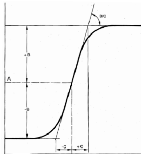
Рис. 1 – Крива функції гіперболічного тангенсу Олدفілда [8]
