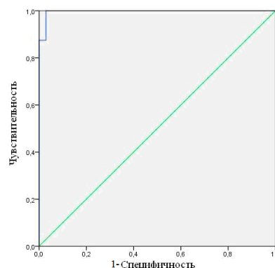
Рис. 1 – ROC-Кривая
