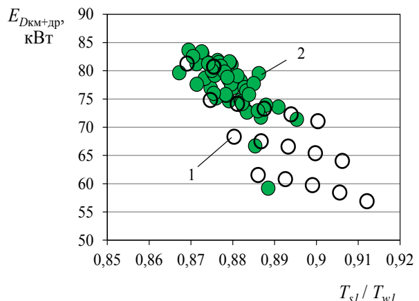
Рис. 16 – Залежність сумарної деструкції ексергії у компресорі і дроселі від T_{s1}/T_{w1} : 1 – еталонний режим; 2 – діагностуємый режим
