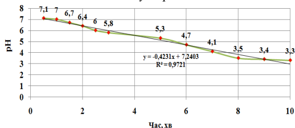
Рис. 3 – Залежність зміни рН аноліту від часу обробки на діафрагмовому електролізері.
