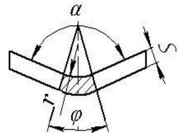
Рис. 1. Угол гибки
