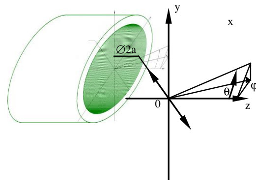
Рис. – Система координат в раскрытии круглого гофрированного волновода
