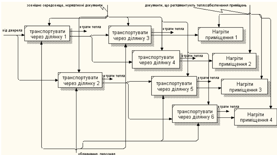
Рис. 3. Функціональна структура СТРТ
