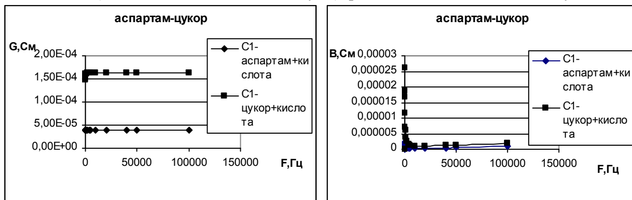
Рис.3. Залежність активної G та реактивної B складових адмітансу від частоти для еквівалентного вмісту цукру та аспартаму у їх кисло-водних розчинах: а) активна складова адмітансу; б) реактивна складова адмітансу.
