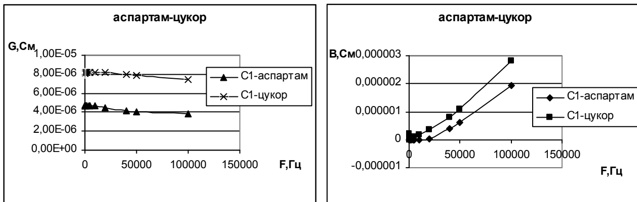
Рис.2. Залежність активної G та реактивної B складових адмітансу від частоти для еквівалентного вмісту цукру та аспартаму у їх водних розчинах: а) активна складова адмітансу; б) реактивна складова адмітансу.
