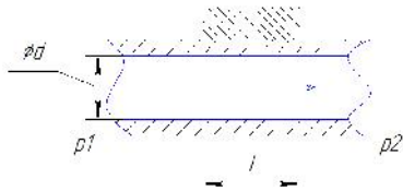
Рис. 2. Рух газу крізь вимірювальну камеру за відсутності сконденсованих компонентів.
