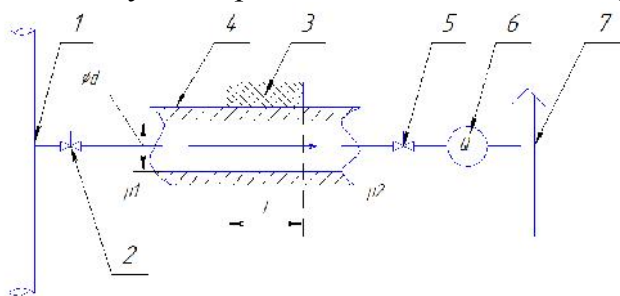
Рис. 1. Схематичний вигляд вимірювального газопроводу
