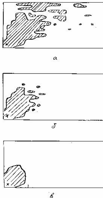
Рис.1. Зоны опасного излучения источника ЭМП электрического типа при различной проводимости стен а - \sigma = 0,2 \text{ См/м} ; б - \sigma = 0,05 \text{ См/м} ; в - \sigma = 0,005 \text{ См/м}
