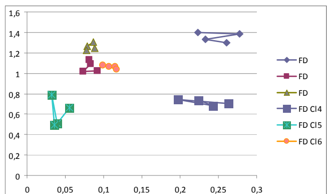
Рис. 4. Залежність складності від варіабельності коливань СР (значення фрактальної розмірності від коефіцієнту варіації) для кожного з кластерів при кожному з інтервалів спостереження
