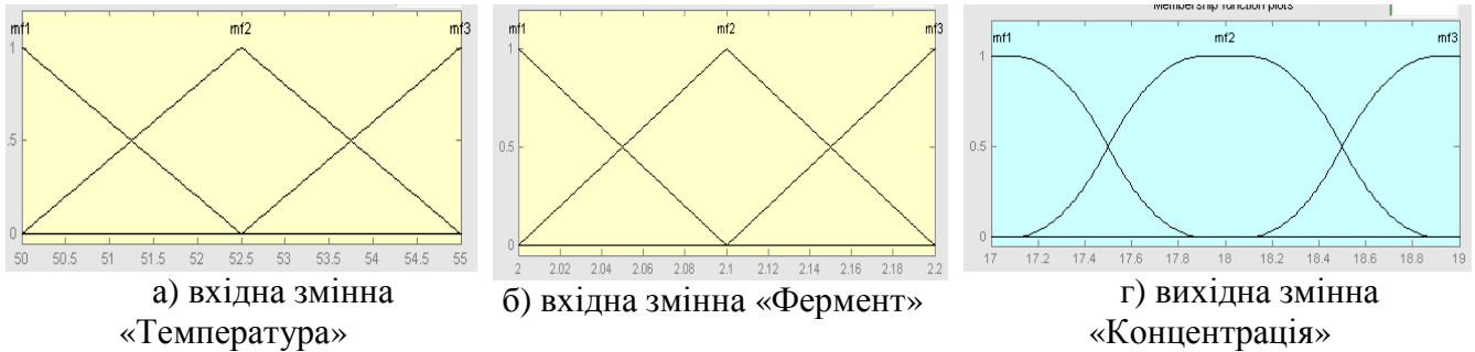
Рис. 2. Функції приналежності
