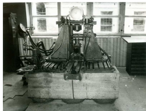
Рис. 1. Вибрационная установка для обработки деталей, выполненная по первому варианту
