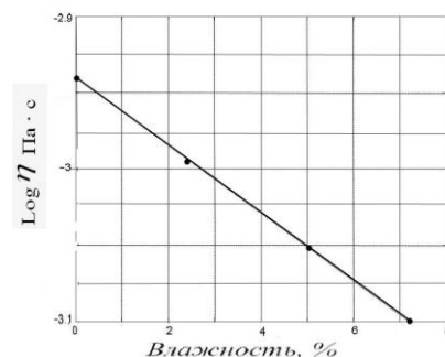
Рис. 1. Зависимость эффективной вязкости от влажности ДПК при \sigma = 4,89 * 10^4 \text{ c}^{-1}
