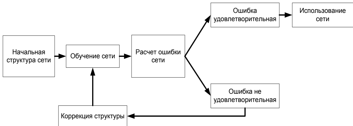
Рис.2- Блок-схема алгоритма построения сети.
