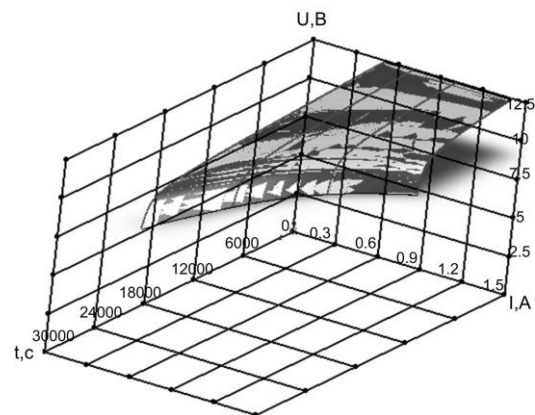
Рис. 3- Разрядная характеристика свинцового аккумулятора.
